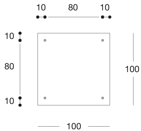
DETTAGLI VISTA FRONTALE (identica per tutti i pannelli) DETAILED FRONT VIEW (same for all panels)
