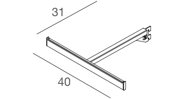
WSBAP2 Barra appenderia piccola in metallo con antisbandieramento Small metal crossbar with anti-swing system L.40 x P. 31 cm
