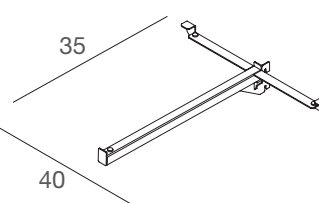
WSRMM/V Staffa reggimensola in metallo per mensola in vetro media, con sistema antisbandieramento Metal bracket for medium glass shelf, with anti- swing system L.40 x P.35 cm
