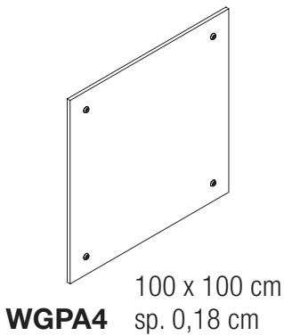
PANNELLO IN NOBILITATO SP.18 mm CON 4 BOCCOLE CHIPBOARD PANEL TH.18 mm WITH 4 PLUGS
