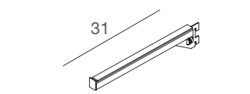
WSAPF Appendiera frontale dritta in metallo con antisbandieramento Metal straight front arm with anti-swing system L.31 cm
