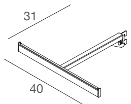
WSBAP2 Barra appenderia piccola in metallo con antisbandieramento Small metal crossbar with anti-swing system L.40 x P. 31 cm
