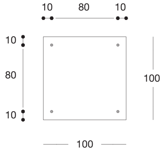
DETTAGLI VISTA FRONTALE (identica per tutti i pannelli) DETAILED FRONT VIEW (same for all panels)
