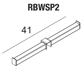
appenderia frontale doppia da applicare su BWSP1-5-15 double frontal hanging bar for RBWSP1-5-15
