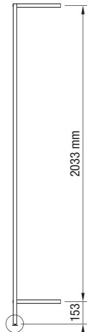
RBWSPM montante in metallo con cremagliera posteriore metal upright with rack on the back
