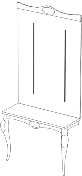
8CONS1 con cremagliere in alluminio grezzo with raw alu racks L125 x P55 x H230 cm
