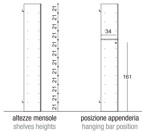
montante centrale middle upright
