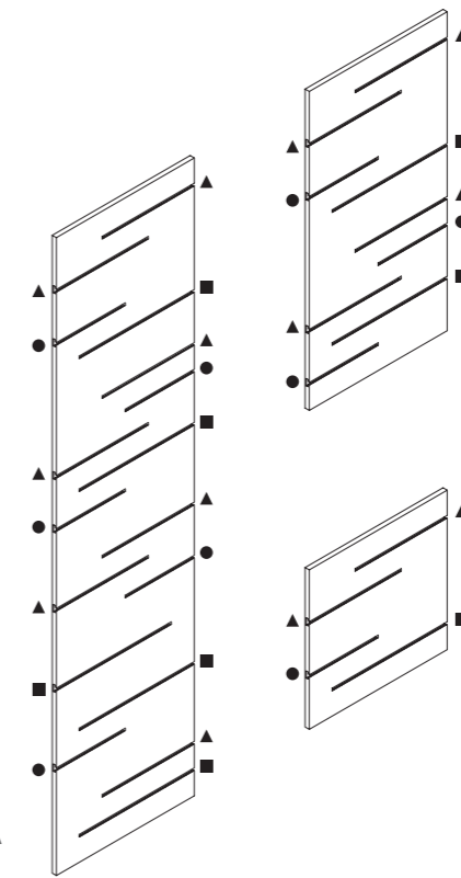
DGT60A L60 x H240 x P1,9 cm
