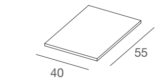
DGMEM mensola in nobilitato chipboard shelf L55 x P40 x SP1,8 cm
