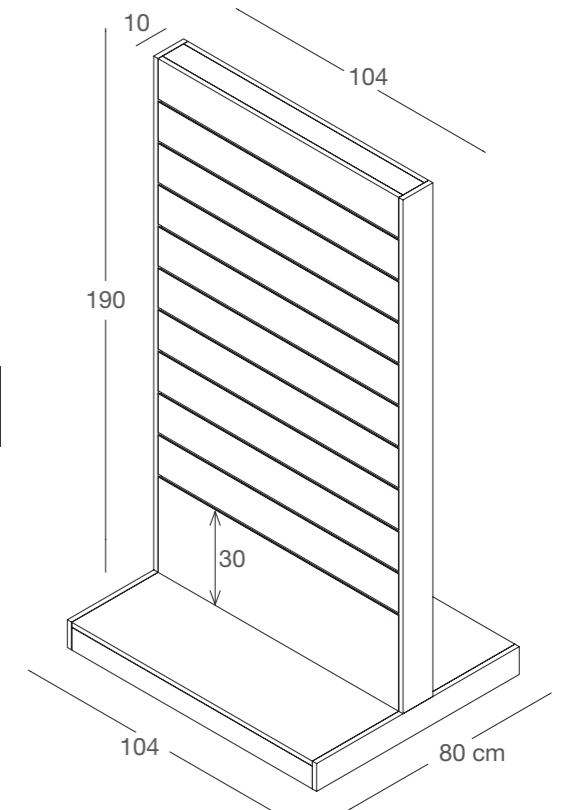
DGFV espositore retro vetrina in nobilitato chipboard display for shop window L104 x P80 x H190 cm
