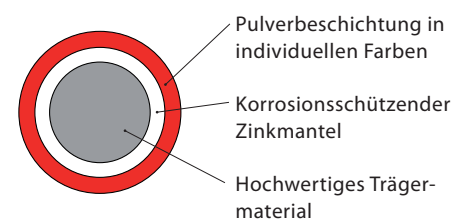
Querschnitt MevoRainbow®
